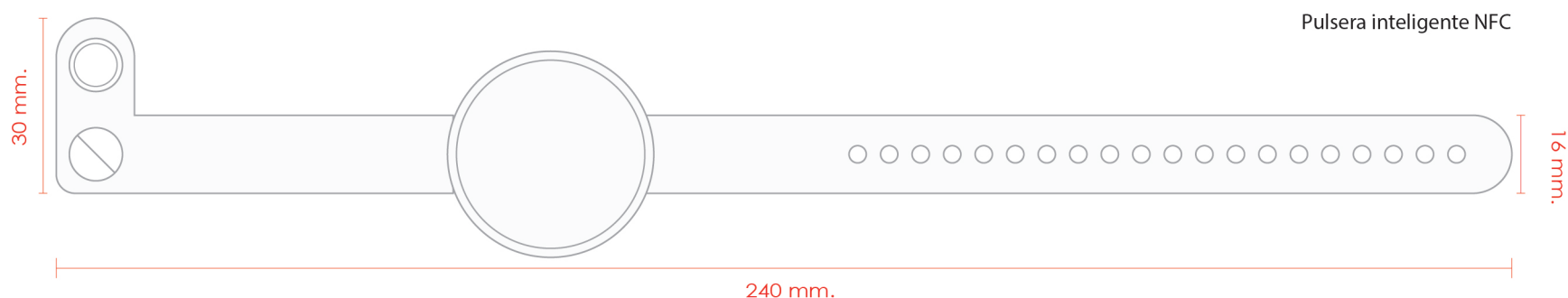
Tag NFC
